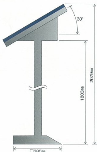
ソーラーパネル外形寸法
