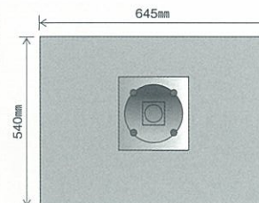
ソーラー面 外形寸法
