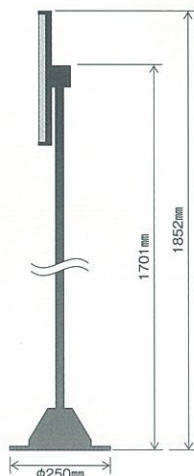
LED照明外形寸法
